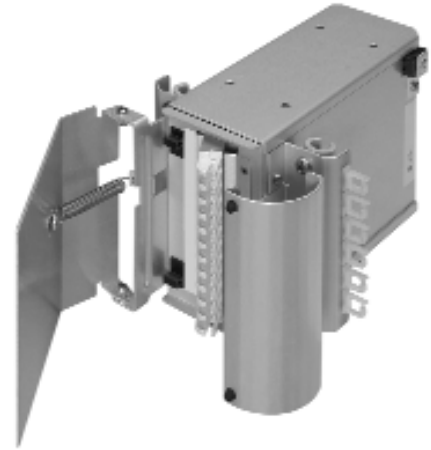
PROFIL value-added splitter module
